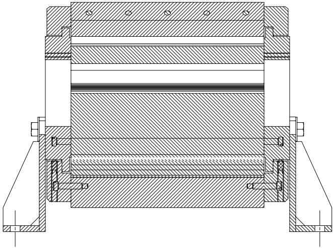
SECTION "A-A" SCALE: FULL
